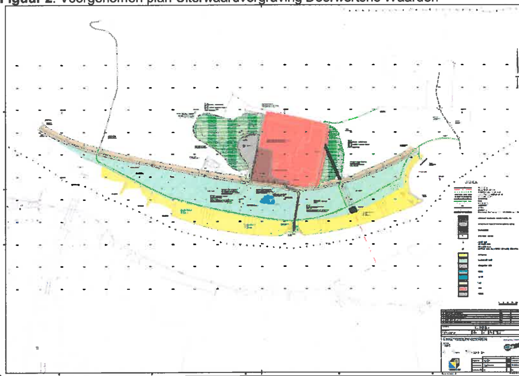
Figuur 2: Voorgenomen plan Uiterwaardvergraving Doorwerthse Waarden
